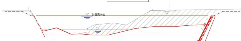
標準断面図
