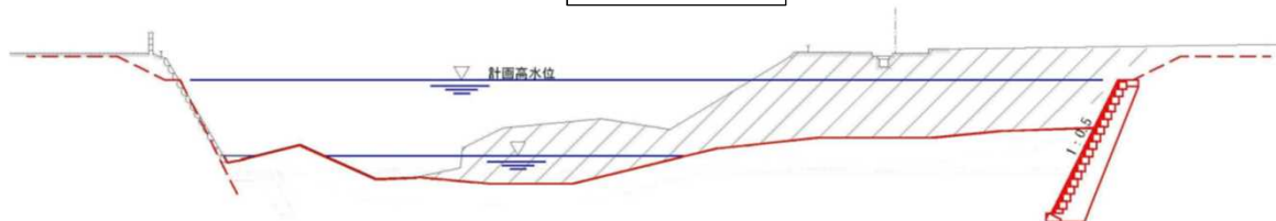
標準断面図
