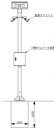
カメラ詳細図
