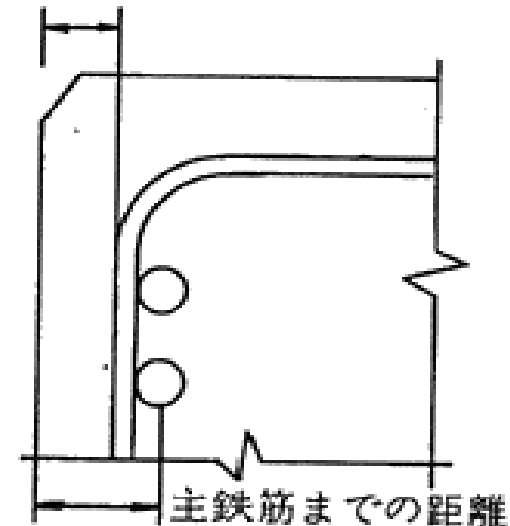
鉄筋のかぶり
