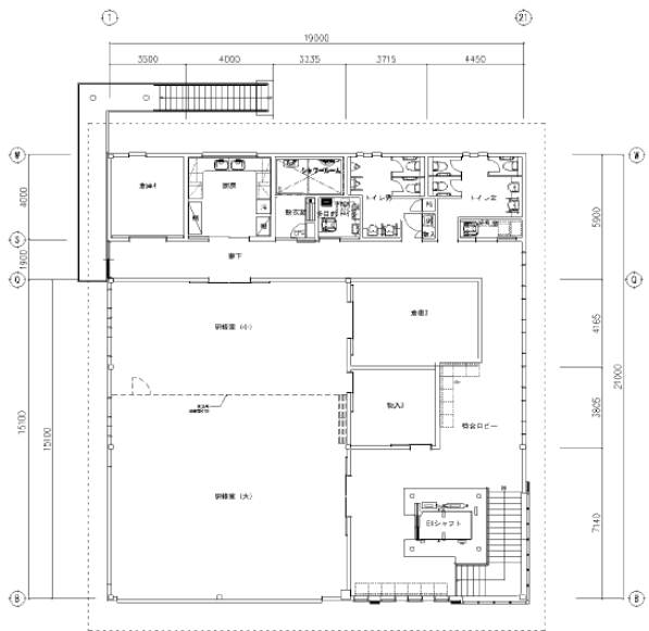
2階平面詳細図 1:100
