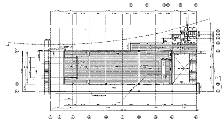
1 全体平面図 SCALE 1:100
