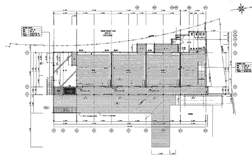
1 廊下平面図 SCALE 1:100
