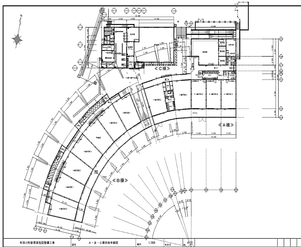
有田川町新保育施設整備工事 図名 A・B・C棟全体平面図 縮尺 1/200 年月日 11/11
