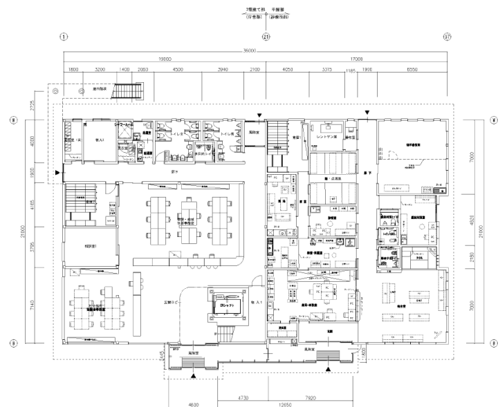
1階平面詳細図 1:100
