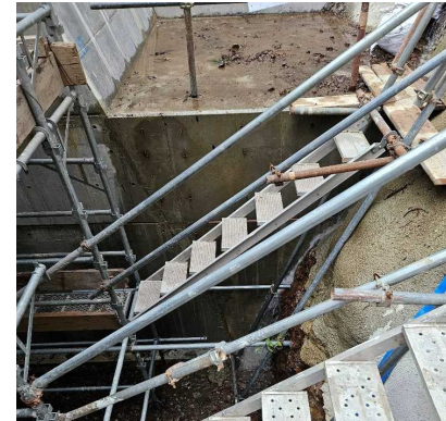
架設通路設置（間詰コンクリート部）
