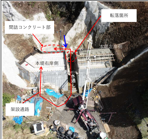
被災前の状況（現場全体）
