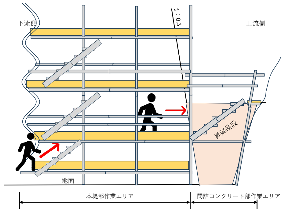
改善対策（架設通路）イメージ図
