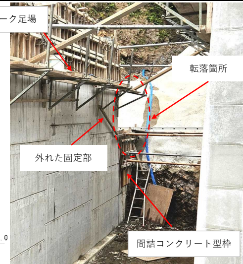
被災後の状況（水通し部）
