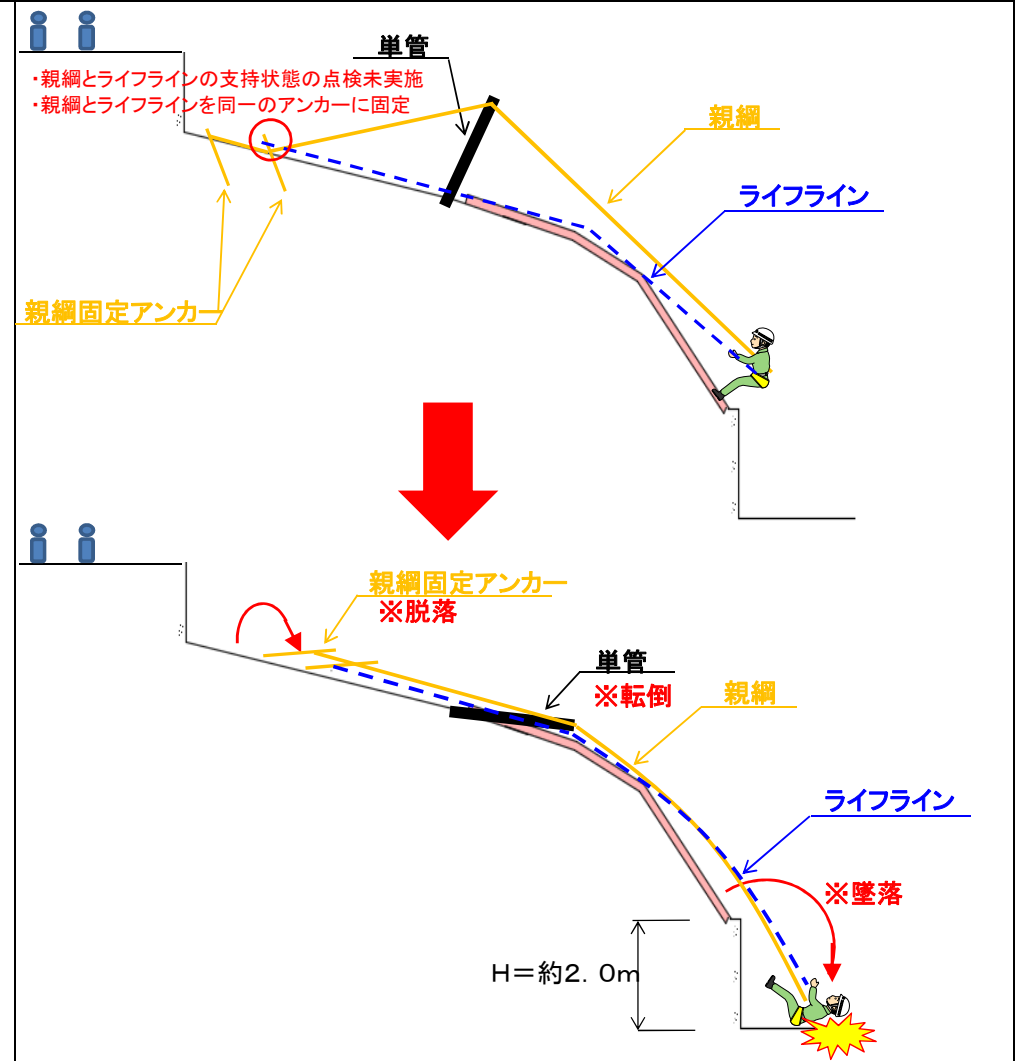
添付資料③-2 : 事故状況断面図
