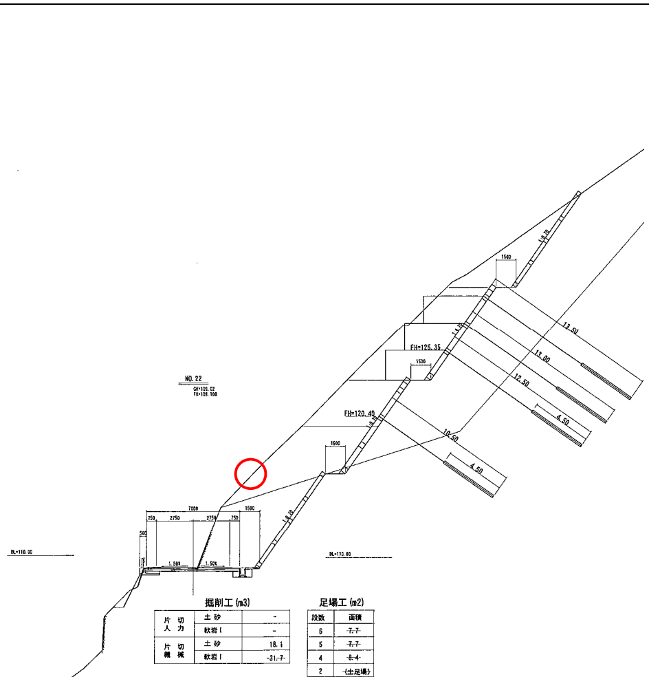
添付資料③—2：事故状況断面図
