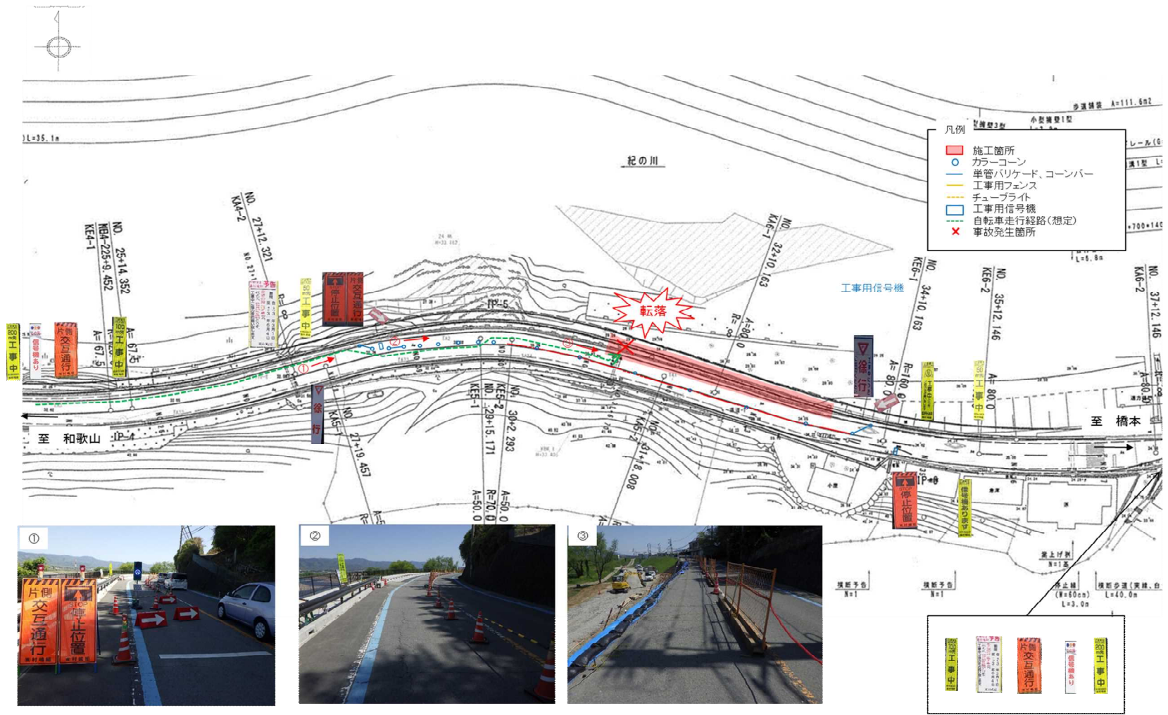
和歌山橋本線（紀の川市竹房）平面図
