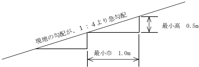
図1-2-1 盛土基礎地盤の段切
