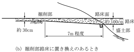
図1-2-3 掘削（切土）部、盛土部接続部のすり付け
