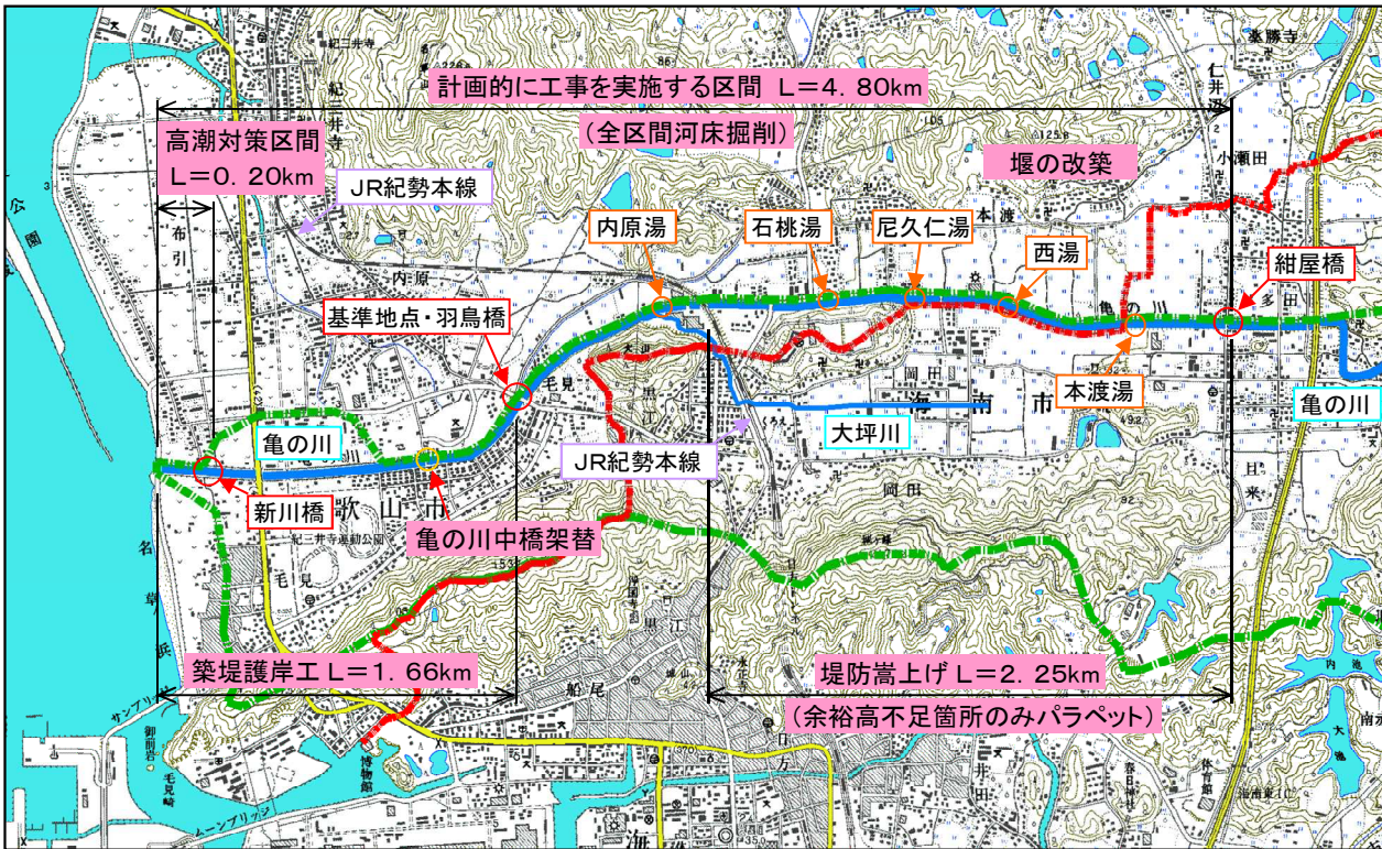
図 5 亀の川河川改修の概要
