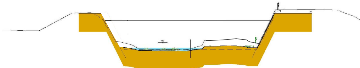
図 6 亀の川改修区間標準断面図
