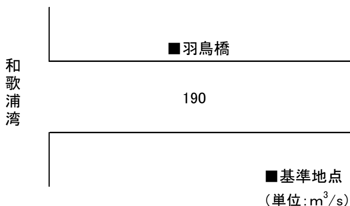
図 4 計画流量配分
