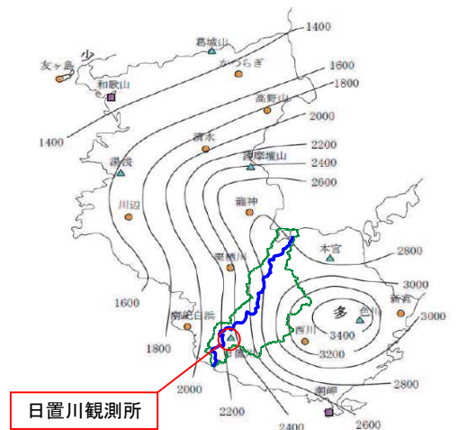
図4 年平均降水量分布図
