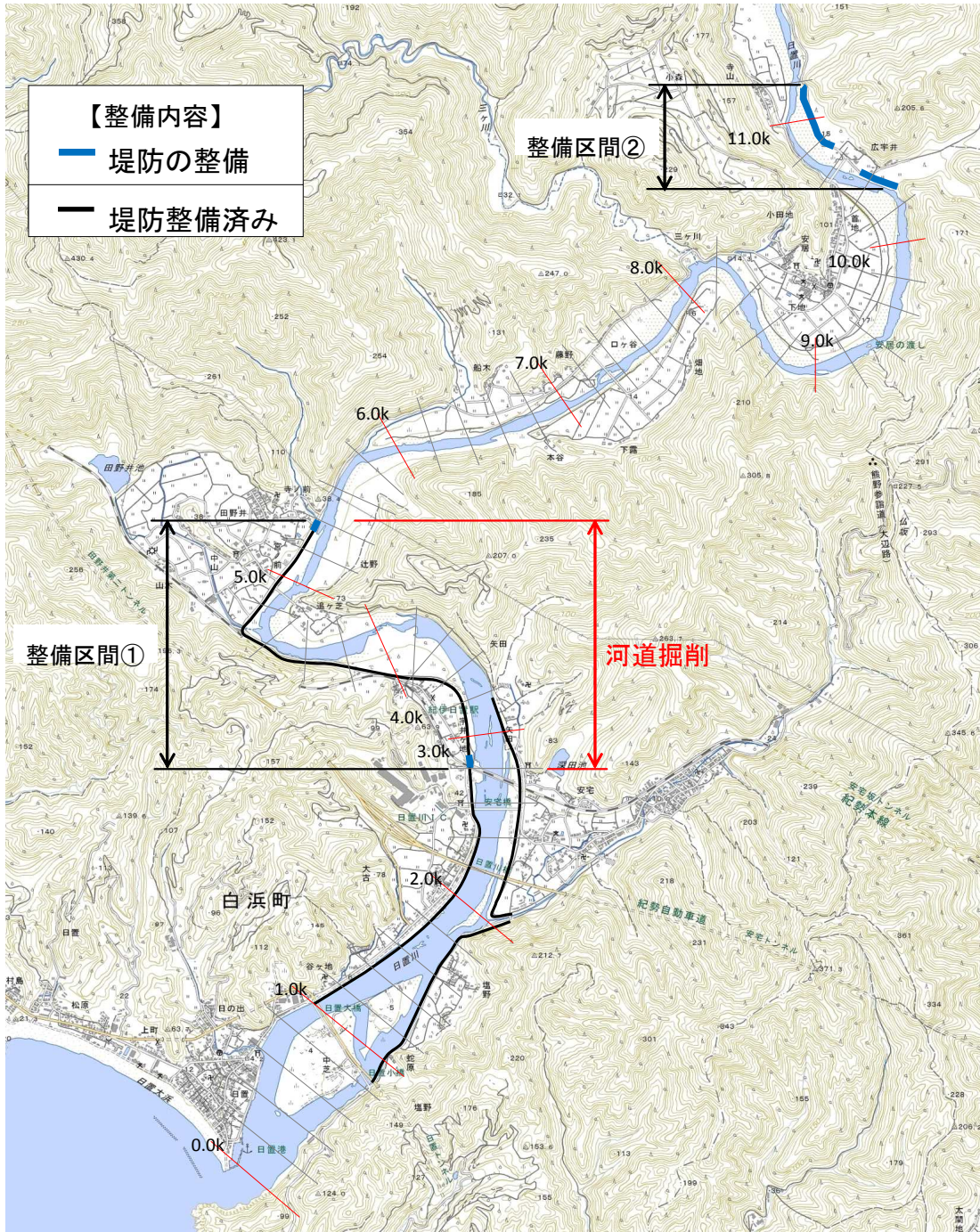
図 1 3 計画的に河川工事を実施する区間
