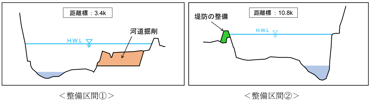
図 1 4 代表横断面図
