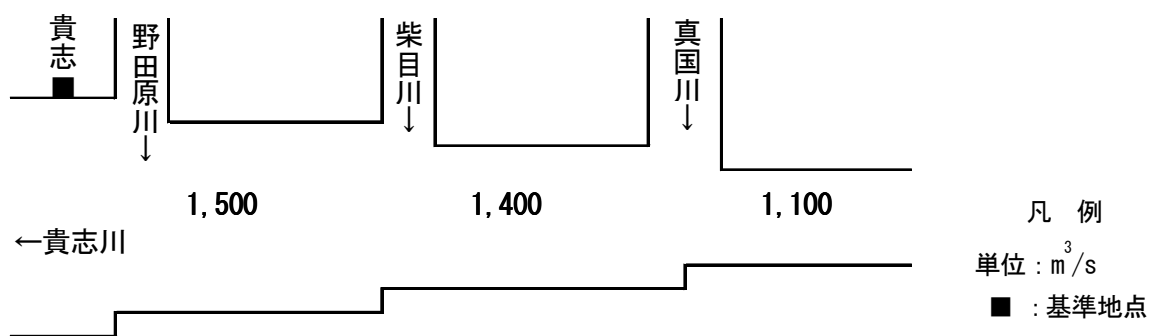
図 18 紀の川水系貴志川圏域河川整備計画目標流量配分図
