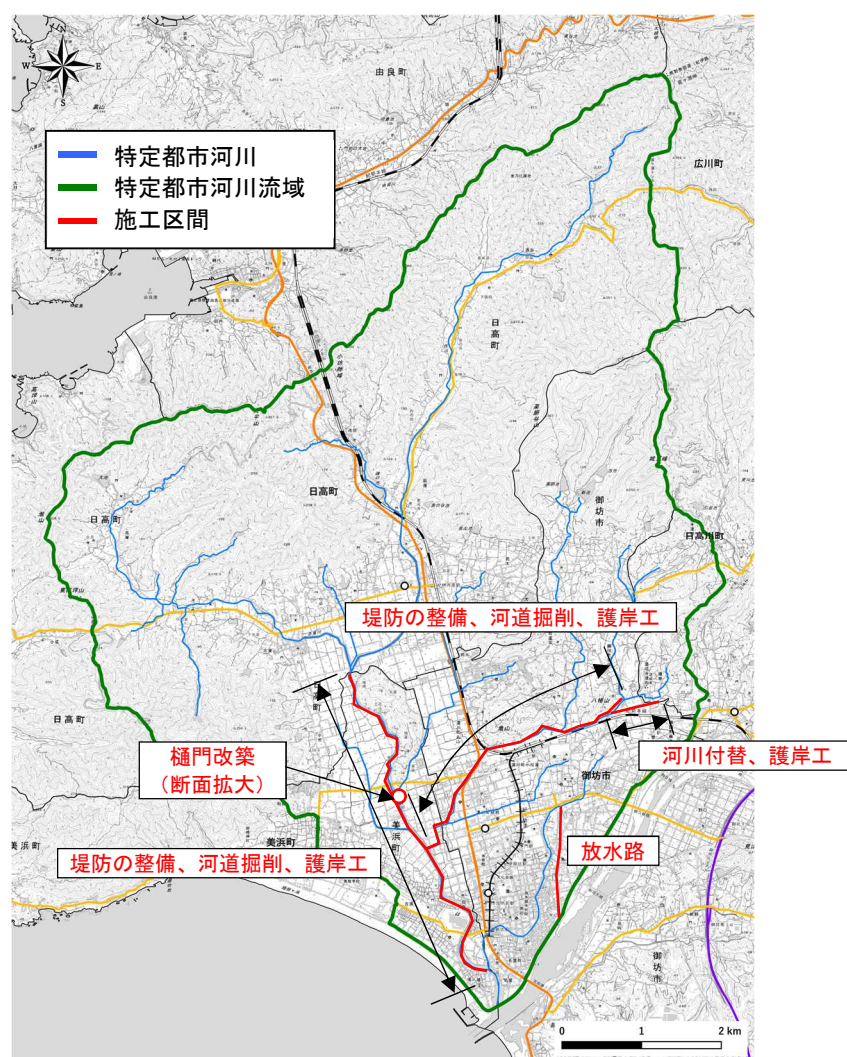
図4-1 河川工事の施工の場所
