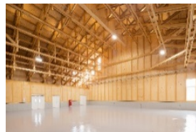
ドクターヘリ格納庫
