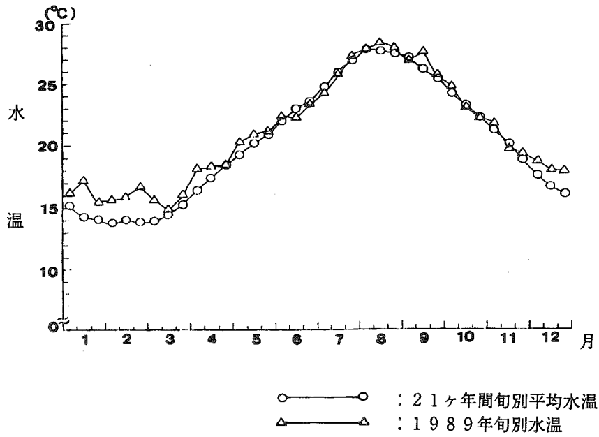
図2 1989年旬別水温と過去21ヶ年間旬別平均水温
