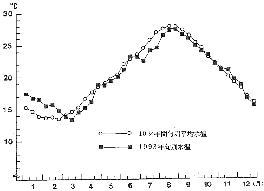
図2 1993年旬別水温と過去10ヶ年間（'83～'92）旬別平均水温
