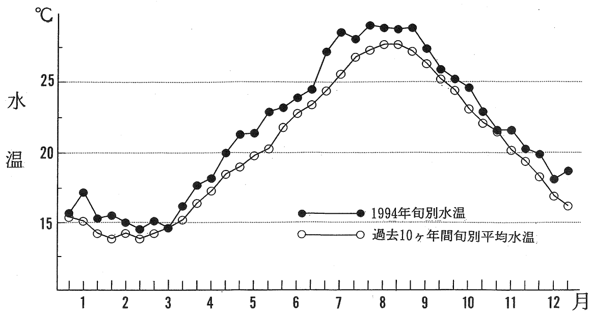
図2 1994年旬別水温と過去10ヶ年間（'84～'93）旬別平均水温
