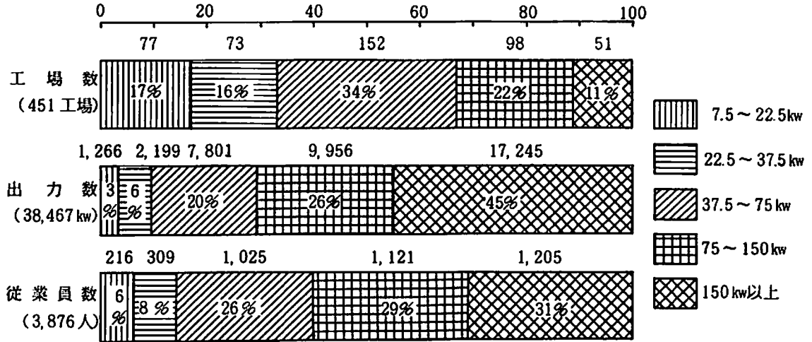
製材工場数等 (56年)
