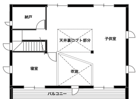
【2階】
