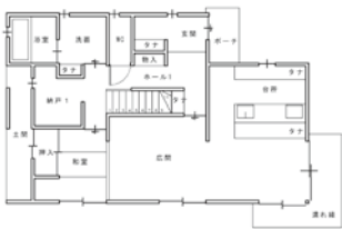
【1階】
