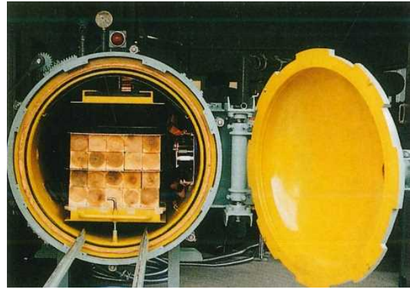
木材乾燥試験 (高周波減圧乾燥機)
