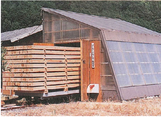
太陽熱利用木材乾燥室による柱材の乾燥試験
