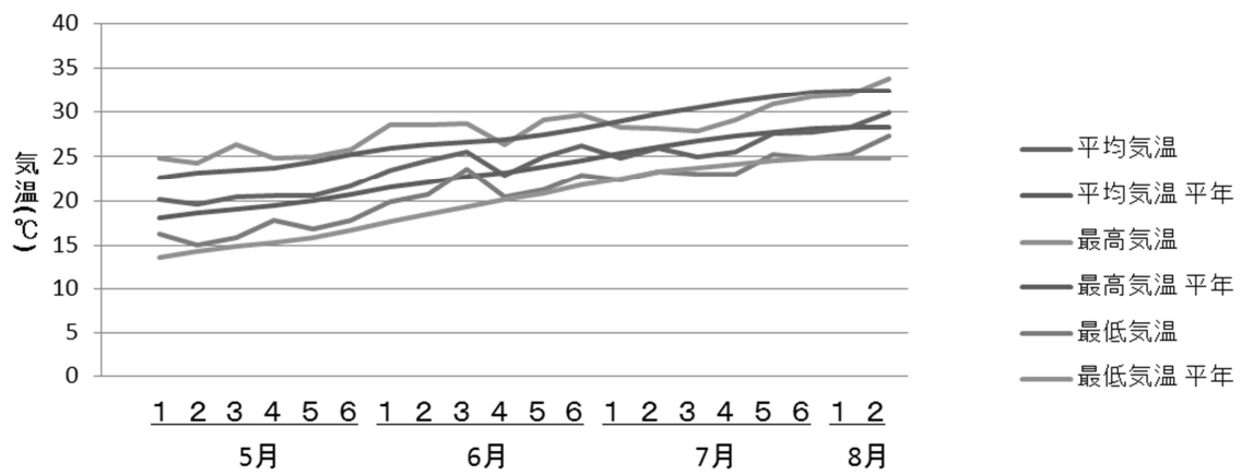
半旬別気温の推移(2020)
