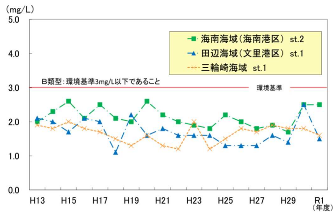
図 3-4-7 COD（化学的酸素要求量）経年変化（75%値）
