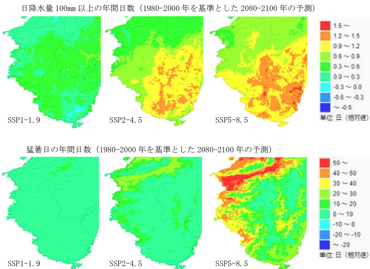
図 3-1-8 将来気候と現在気候の変化分布図
