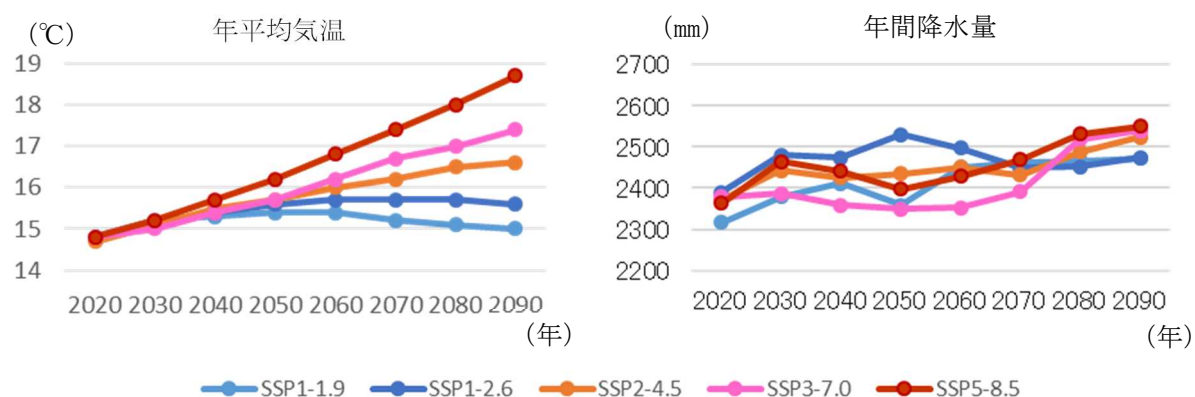
図 3-1-7 本県の年平均気温及び年間降水量の将来予測
