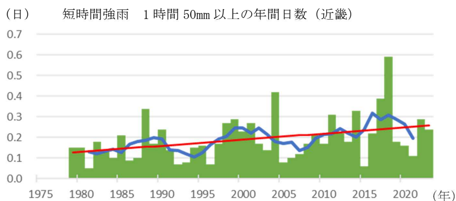
図 3-1-5 近畿地方のアメダス 1 地点当たりの短時間強雨（1 時間降雨量 50 mm 以上）の発生回数の変化（出典：気象庁 HP）
