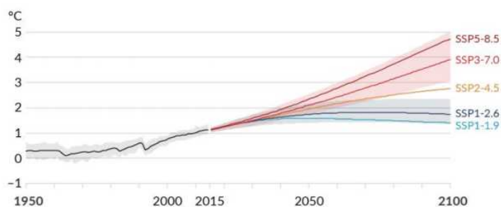
図 3-1-2 1850～1900 年を基準とした世界平均気温の変化
