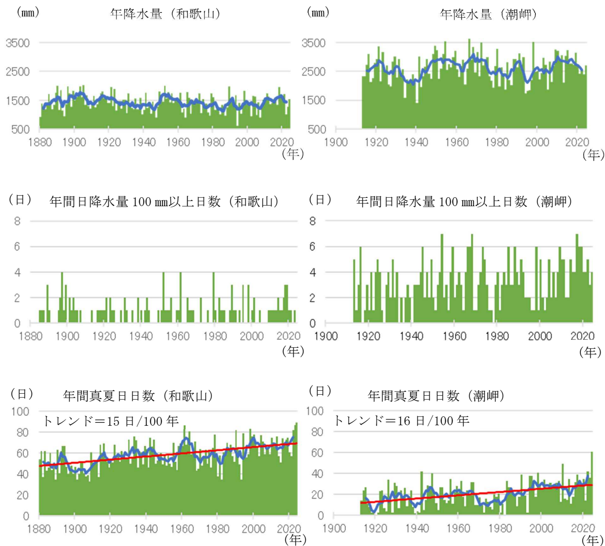
図 3-1-4 本県（和歌山地方気象台・潮岬）の気象状況の変化（出典：気象庁 HP）（続き）
