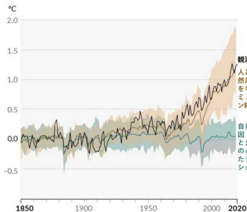
図 3-1-1 世界平均気温の観測値とシミュレーション
