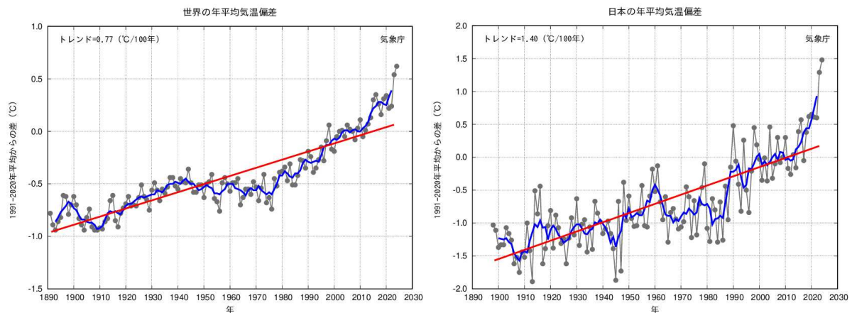
図 3-1-3 世界の年平均気温偏差の経年変化（左） 日本の年平均気温偏差の経年変化（右）※ 1 （出典：気候変動適応情報プラットフォーム HP、気象庁 HP）
