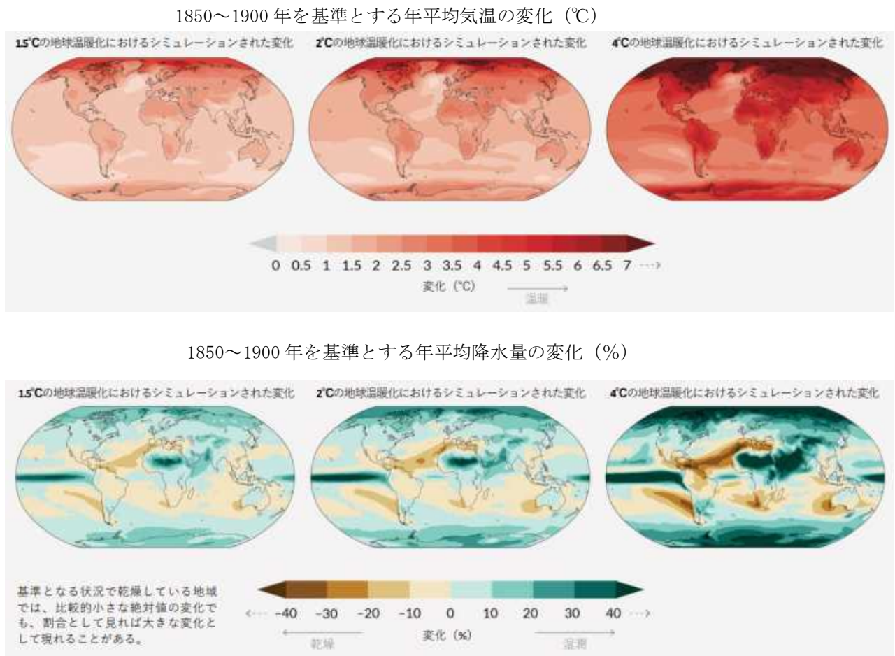
図 3-1-6 1850～1900 年を基準とする 20 年平均の世界平均気温で、1.5℃、2℃及び 4℃の地球温暖化の水準（世界の年平均地上気温変化及び年平均降水量変化）
