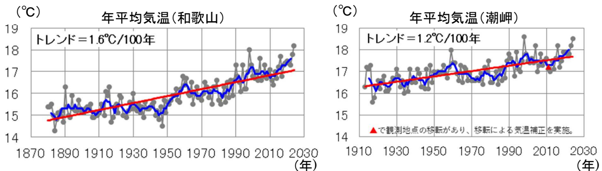
図 3-1-4 本県（和歌山地方気象台・潮岬）の気象状況の変化（出典：気象庁 HP）
