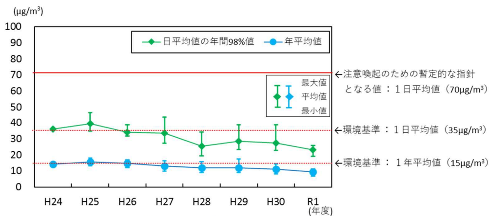
図 3-4-5 PM2.5 (微小粒子状物質) の経年変化 (県内全測定局の平均値)
