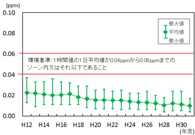
図 3-4-1 二酸化窒素の経年変化 (県内全測定局の日平均値の年間 98%値)
