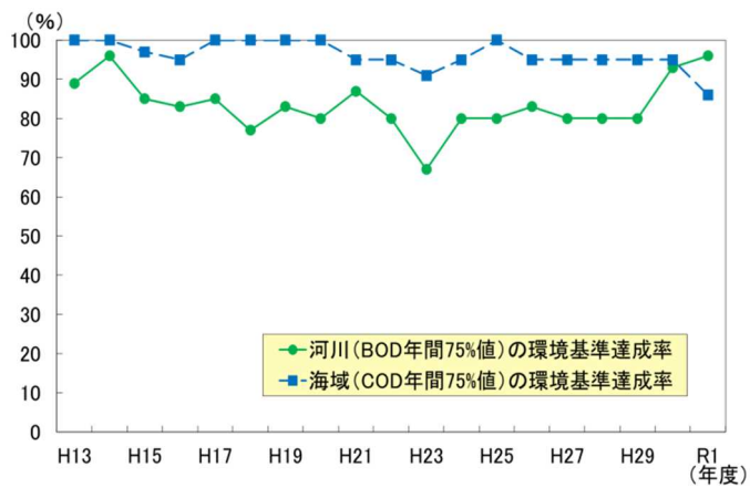
図 3-4-8 河川・海域別環境基準達成率の推移
