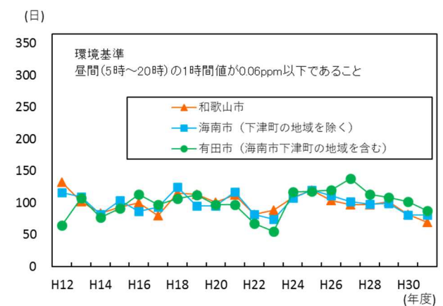
図 3-4-4 光化学オキシダントの環境基準超過 日数の経年変化 (予報等の発令地域別におけ る昼間の1時間値がが環境基準を超過した日数)
