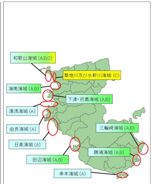
図 3-4-10 海域の COD に係る類型指定状況
