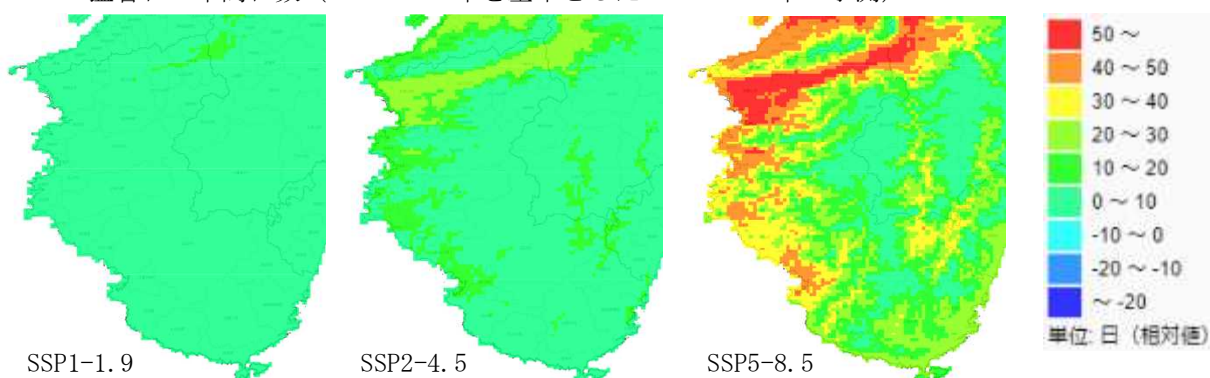
図 3-1-8 将来気候と現在気候の変化分布図
