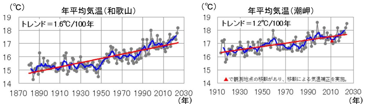
図 3-1-4 本県（和歌山地方气象台・潮岬）の気象状況の変化（出典：気象庁 HP）
