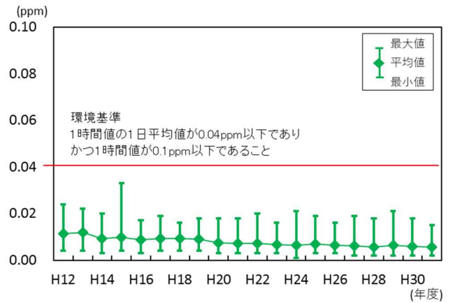
図 3-4-2 二酸化硫黄の経年変化 (県内全測定局の日平均値の 2%除外値)
