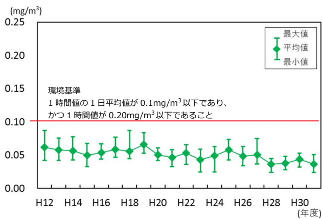
図 3-4-3 浮遊粒子状物質 (SPM) の経年変化 (県内全測定局の日平均値の年間 98%値)
