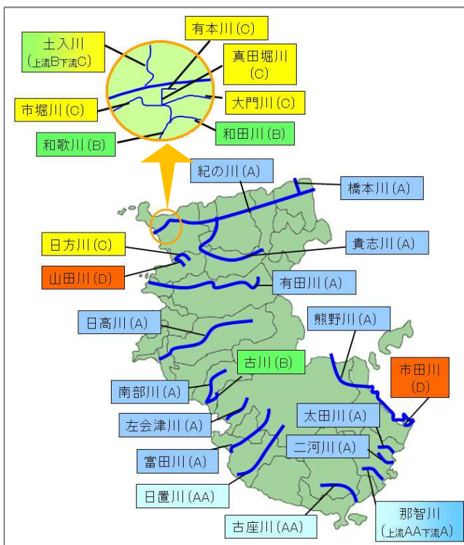
図 3-4-9 河川の BOD に係る類型指定状況
