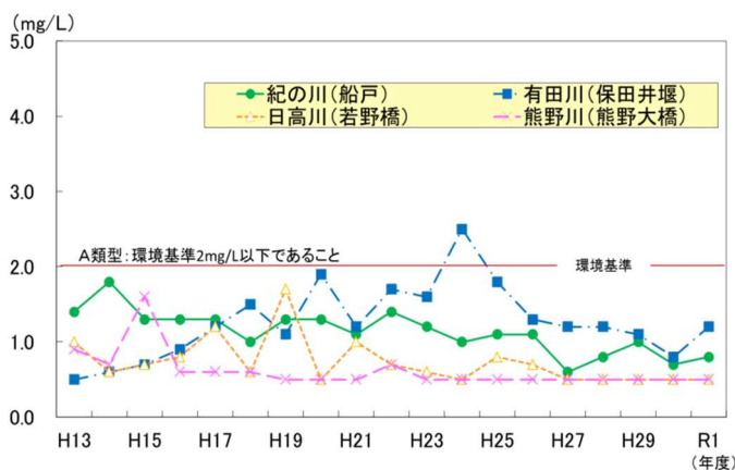
図 3-4-6 BOD（生物化学的酸素要求量）経年変化（75%値）
