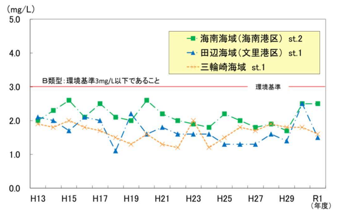
図 3-4-7 COD（化学的酸素要求量）経年変化（75%値）
