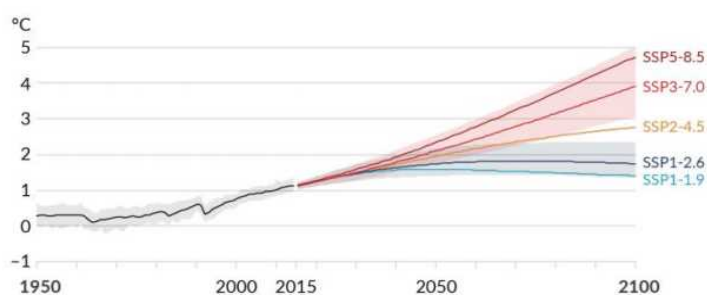
図 3-1-2 1850～1900 年を基準とした世界平均気温の変化
