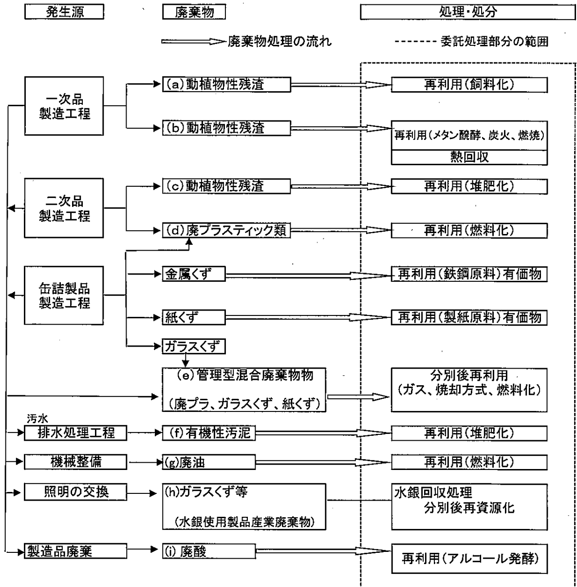
別添ー1. 廃棄物処理フロー図
